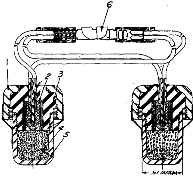
SPOILER ACTUATOR
